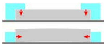
Otočení, hrubování, uvolnění (DEMAG/MAG) a obrábění na čisto 2. plochy
